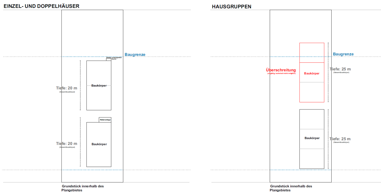
Abbildung 4: schematische Visualisierung zur Regelung der abweichenden Bauweise (unmaßstäbliche Darstellung)
