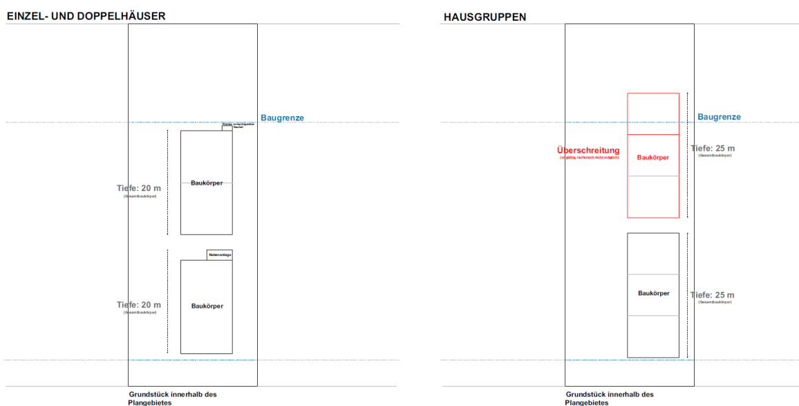
Abbildung 3: schematische Visualisierung zur Regelung der abweichenden Bauweise (unmaßstäbliche Darstellung)
